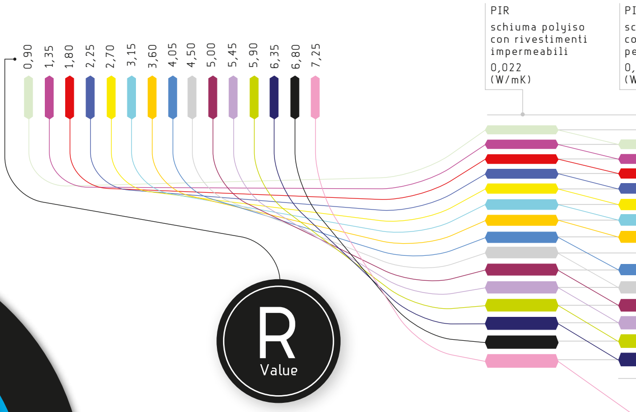
Comparazione spessori a valore costante di resistenza termica
