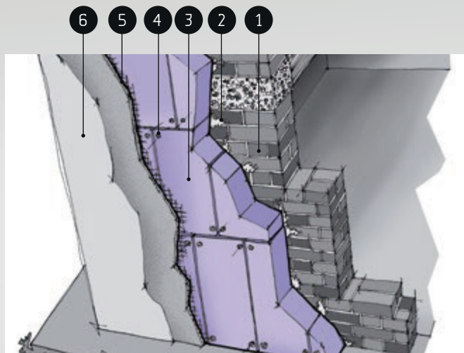
1. MURATURA / 2. COLLANTE CEMENTIZIO / 3. X-FOAM 4. TASSELLI DA CAPPOTTO / 5. RASATURA ARMATA / 6. FINITURA
